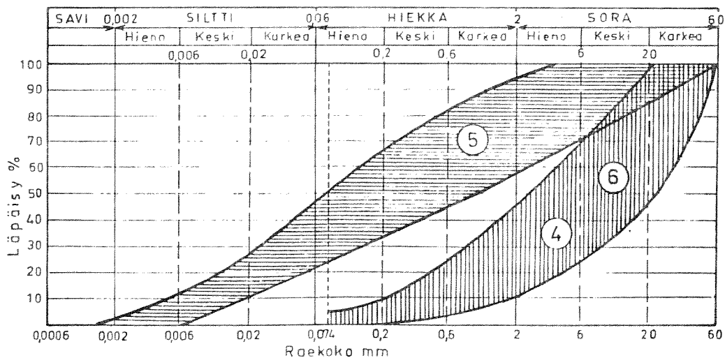
Kuva 3. Vyöhykkeiden rakeisuuden ohjealueet. Moreenirunko (5), suodatin-sora (4,6).
