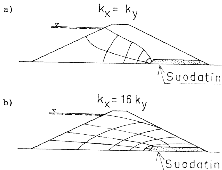
Kuva 16. Virtausverkot läpäisemättömällä pohjalla olevassa maapadossa, a) vaaka- ja pystysuorat vedenläpäisevyyškertoimet yhtä suuria ( k_x = k_y ), b) vaakasuora vedenläpäisevyyškertoimen suurempi kuin pystysuora ( k_x = 16 k_y ).Cedergren 1948.
