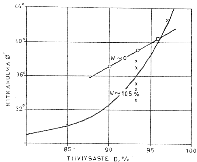
Kuva 28. Hautaperän moreenin tehokkaan kitkakulman \phi' riippuvuus tiiviysasteesta D vesipitoisuuksilla w = 10,5\% ja w = 0\% (suora w = 0 Kotakorpi 1979). Vesipitoisuudet kolmiaksaalikohteiden leikkauksen alussa (cu-kokeet).
