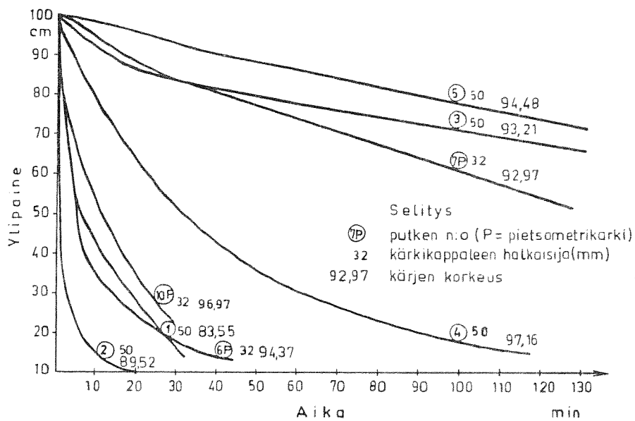
Kuva 15. Hautaperän padon paalun 8+47 vedenläpäisevyyskokeiden mittaustulokset käyrinä.
