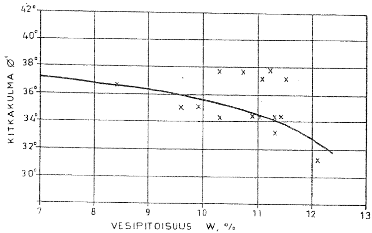
Kuva 27. Hautaperän moreenin tehokkaan kitkakulman \phi' riippuvuus vesipitoisuudesta w , kun tiiviysaste D = 93\% . Vesipitoisuudet kolmiaksaalikohteiden leikkauksen alussa (cu-kokeet).
