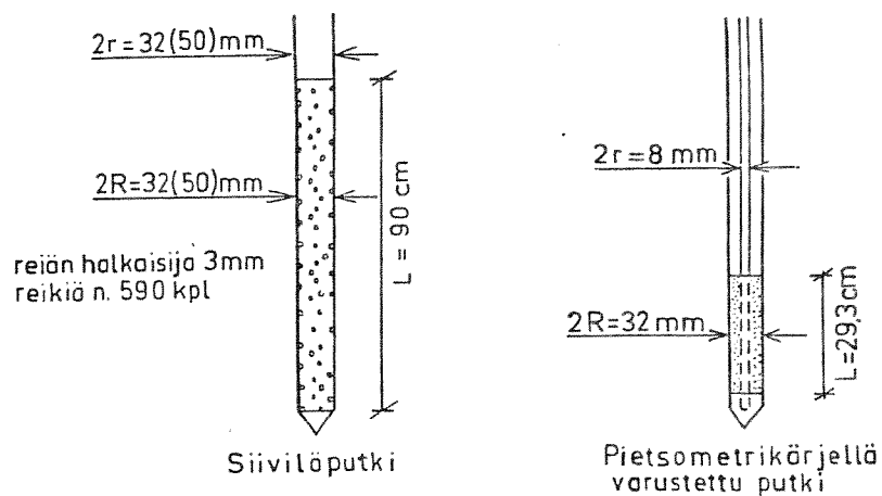
Kuva 14. Hautaperän maapadon vedenläpäisevyyškokeiden 20.-23.6.1977 kaaviokuva.
