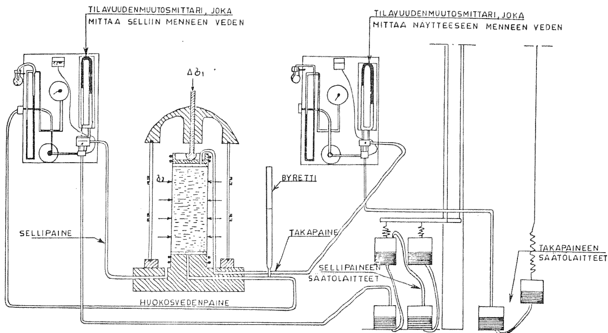
Kuva 22. Kolmiakσιαalisen puristuskokeen laitteiden kytkentäkaavio.
