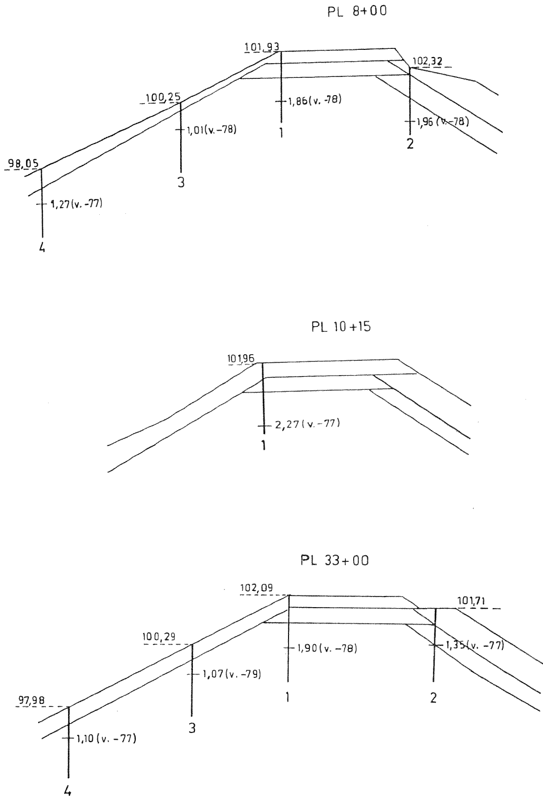
Kuva 12. Suurimmat mitatut routasyvytydet Hautaperän maapadossa vuosina 1977-1980. PL 8+00 mittauksia v. 1977-1978 (v. -78 ei mittari n:o 4). PL 10+15 mittauksia v. 1977. PL 33+00 mittauksia v. 1977 kaikki mittarit, v. 1978 n:ot 1 ja 3, v. 1979-1980 n:o 3.
