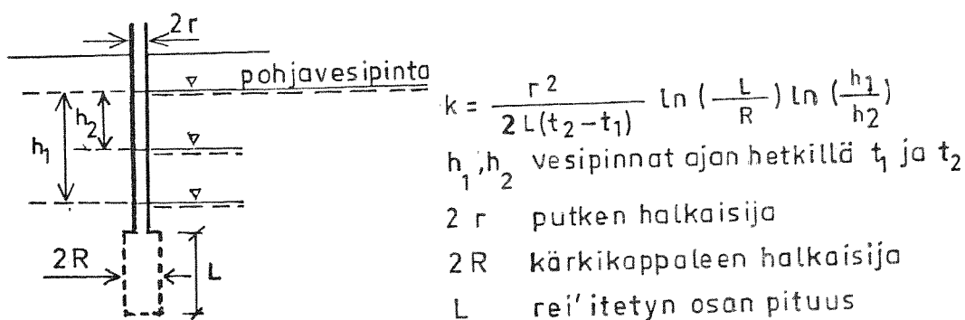
Kuva 13. Vedenläpäisevyyškertoimen määrittäminen.
